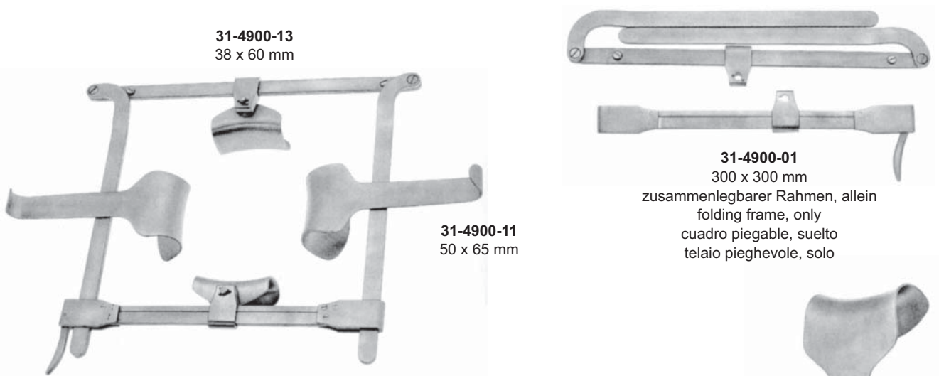
FRANZ 31-4900-00 komplett complete completo completo 1 x 31-4900-01 2 x 31-4900-11 2 x 31-4900-13
